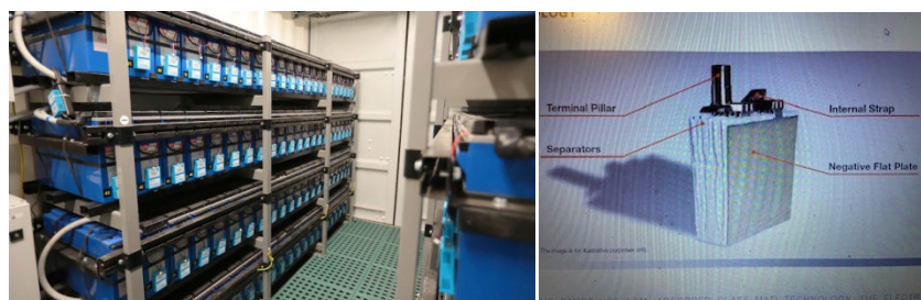
Figuur 2: Kast met accu's, inverter, en een schematische voorstelling van carbon lood met glasplaat.
